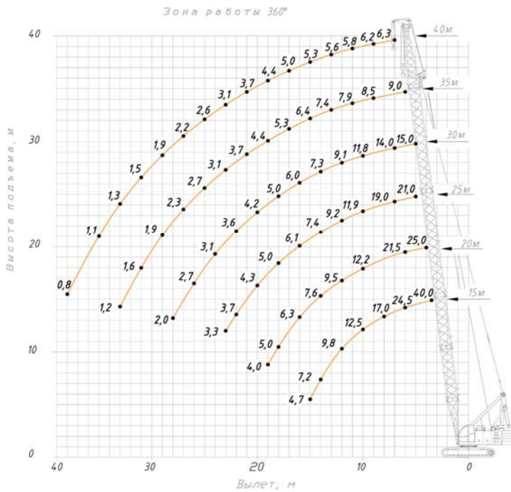
Грузовысотные характеристики основного подъема (вспомогательный гусек не установлен), противовес 14,0 т, угол наклона рабочей площадки \pm 0,5^\circ Зона работы 360°
