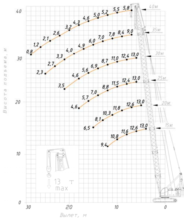
Грузовысотные характеристики вспомогательного подъема (основная стрела 15,0-40,0 м), противовес 14,0 т, угол наклона рабочей площадки \pm 0,5^\circ
